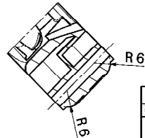
Schnitt-A-A Maßstab: 1:1
