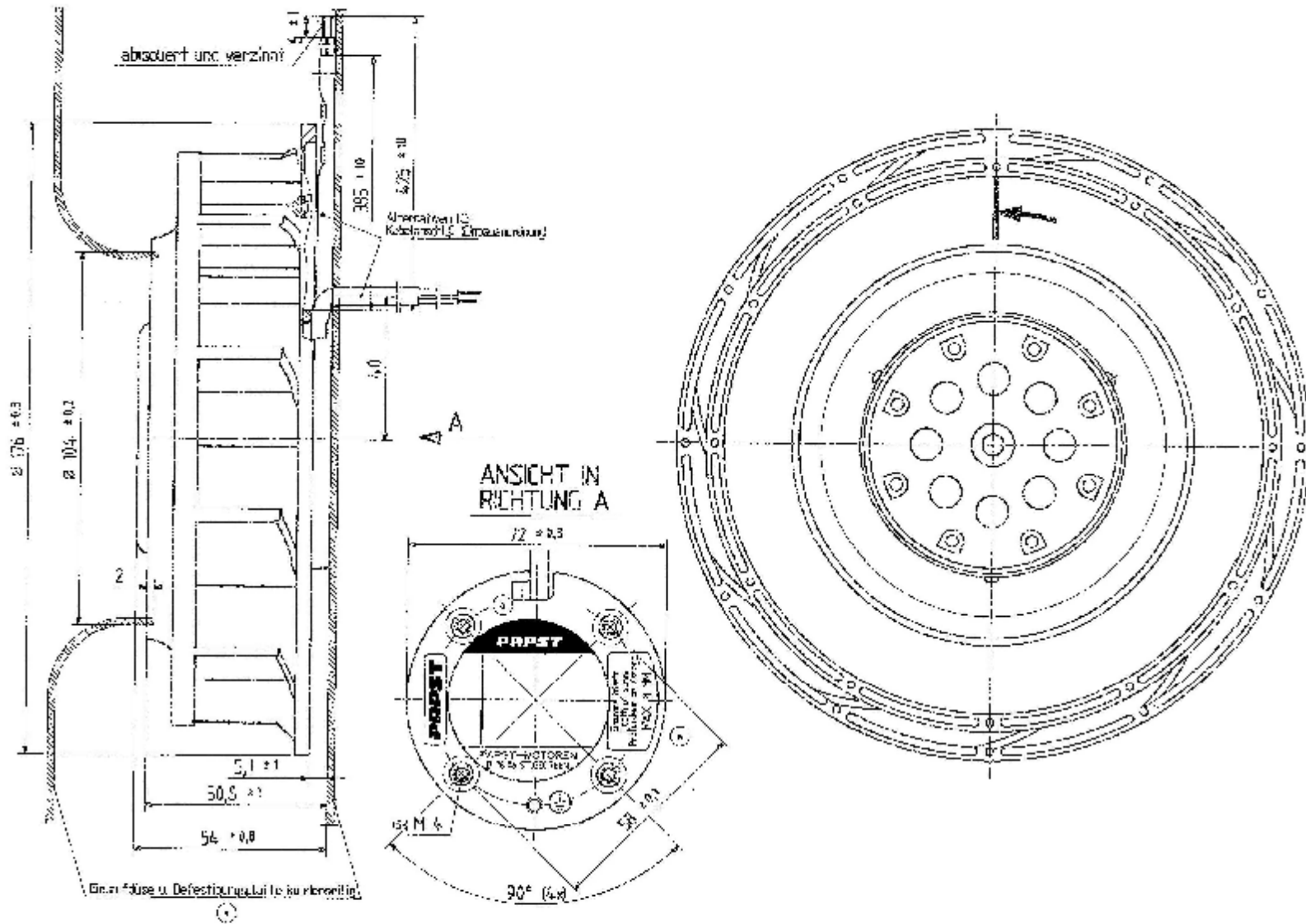
Axialspiel mit Feder spielfrei gespannt
